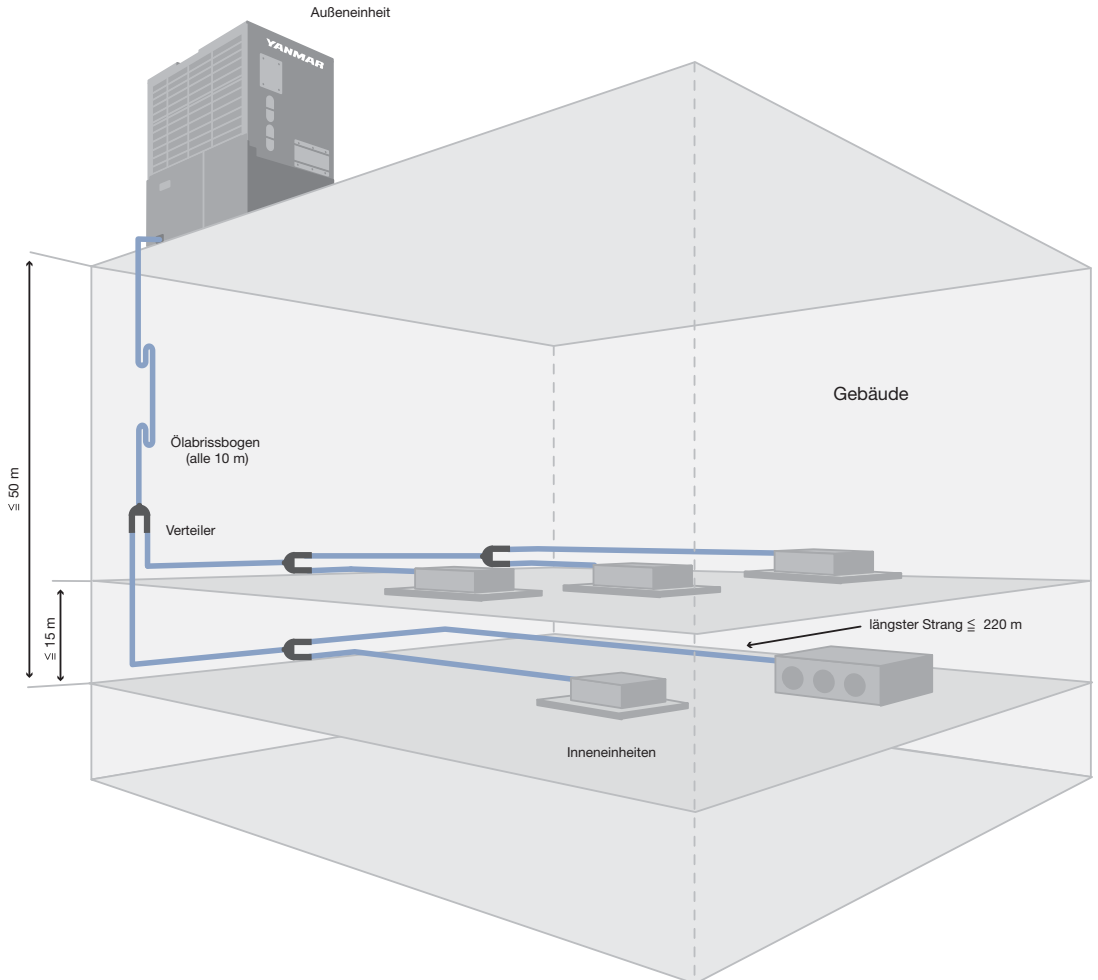
Abb. 3-2 Kältetechnische Grundstruktur einer VRF-Multisplitanlage (Werkbild: Fa. KKU Concept)
