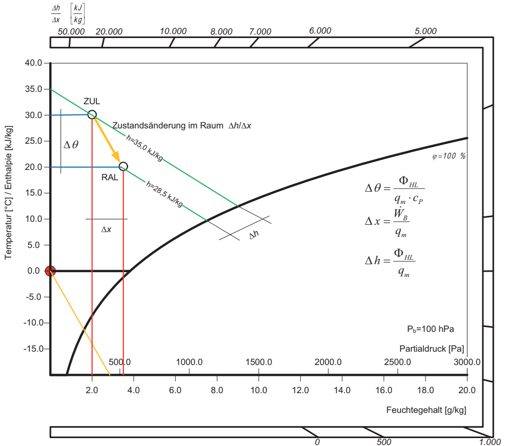
Abb. 2.4-1 Schematische Darstellung der Zustandsänderung im Raum für den Winterfall
